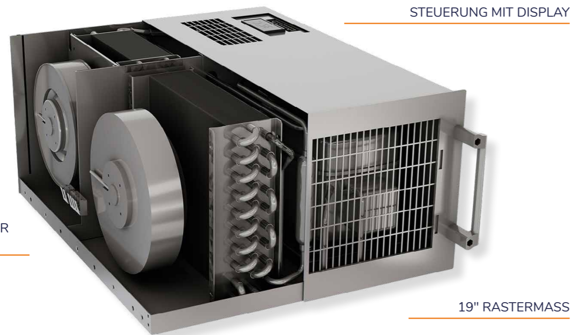
Abb. Kompressorkühlgerät 19"
